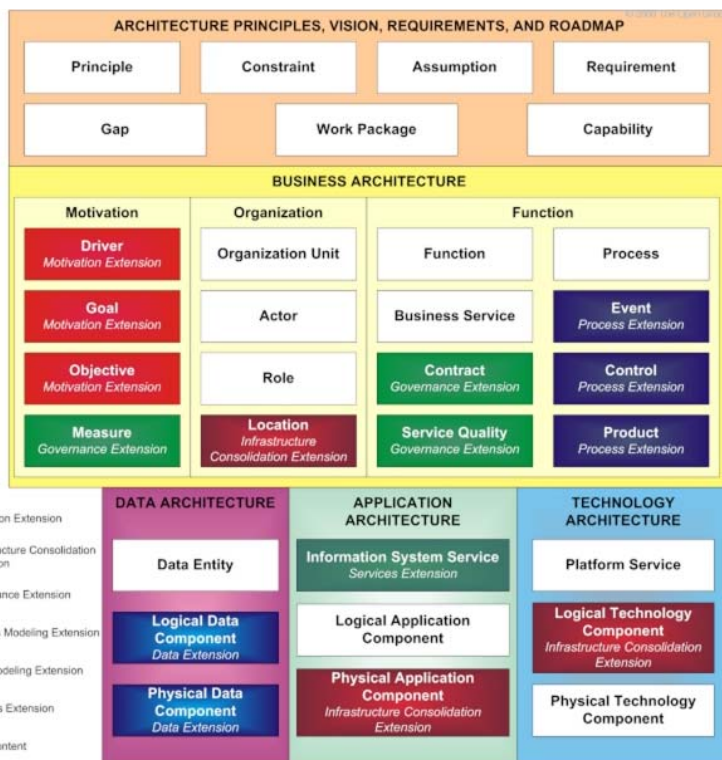
Afbeelding 4: Content metamodel (bouwblokken).
