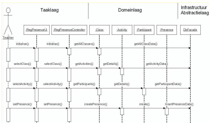
Figuur 3: Sequence diagram bij stap 4 voor de significante use case 'Registreer Aanwezigheid/ Register Presence'. Het gerelateerde lagenmodel is in figuur 1 afgebeeld.
